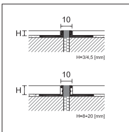
NTA/10 alluminio naturale + EPDM grigio levigabile RAL 7046
